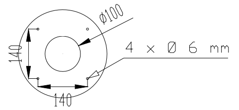
Pletina anclaje a suelo / Floor fixing flange
