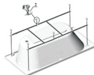
Рисунок 2- Установка кронштейна
